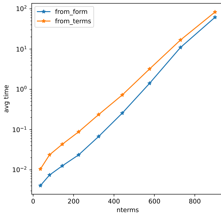
XXZ**2
