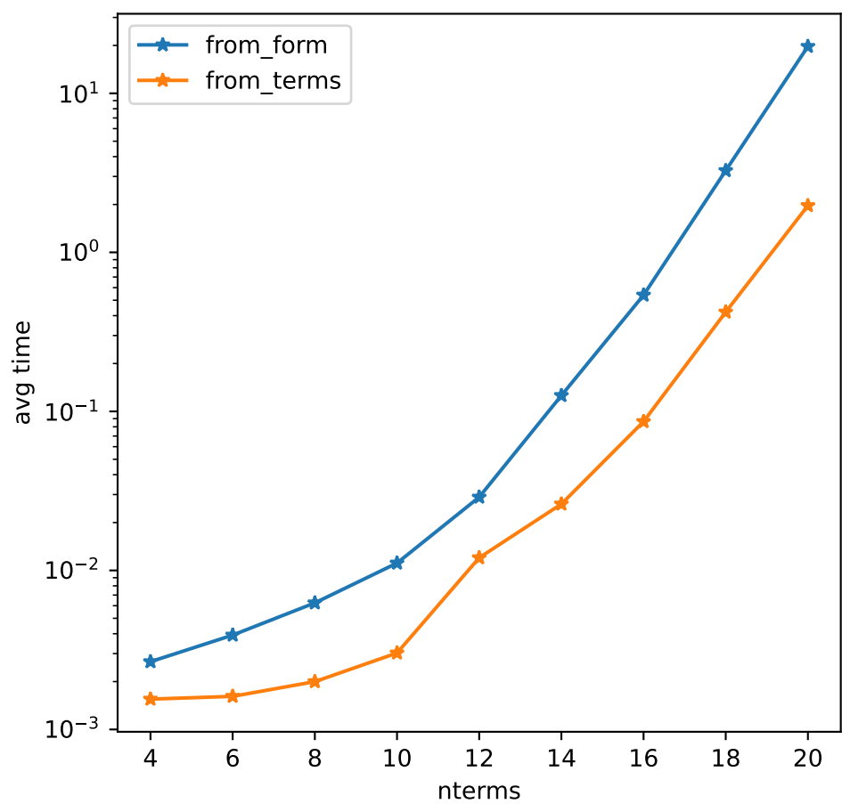
TFIM**2
