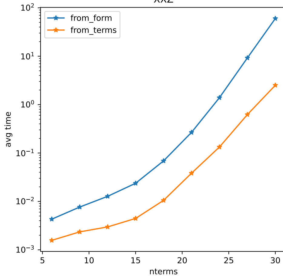
XXZ**2
