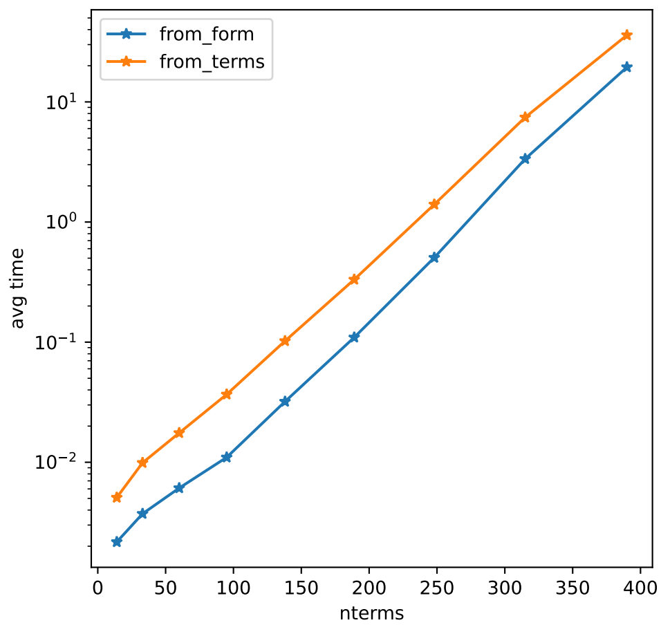
TFIM**2
