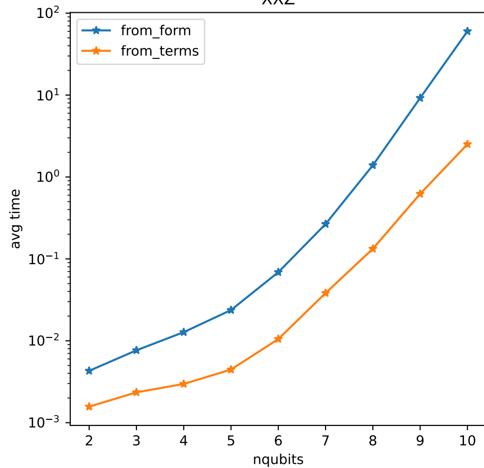
XXZ**2
