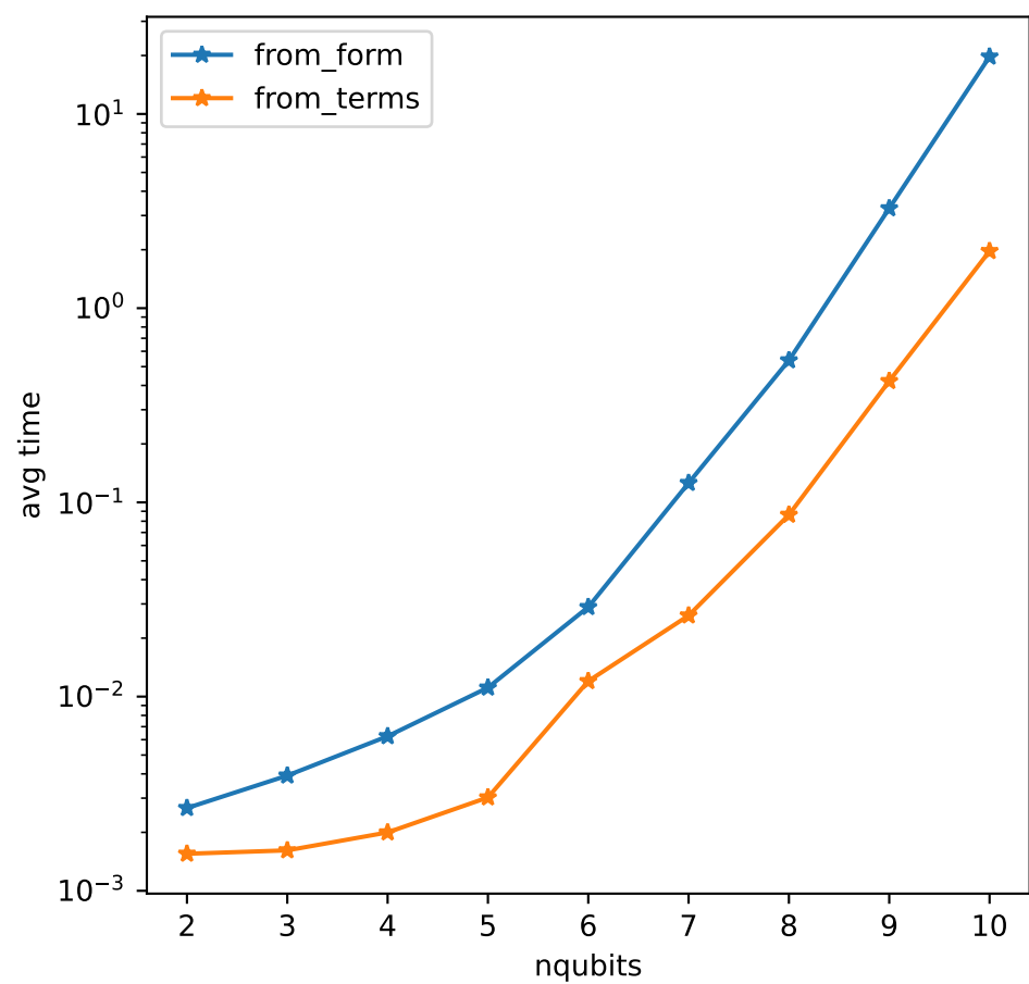
TFIM**2
