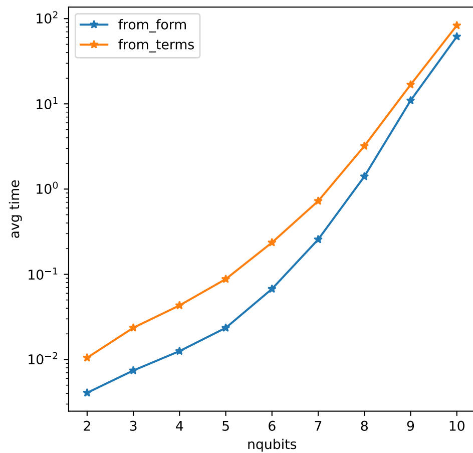
XXZ**2
