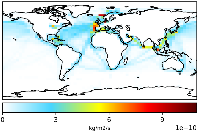
gcc_carbon-CO2 (Ref) 4.0x5.0
