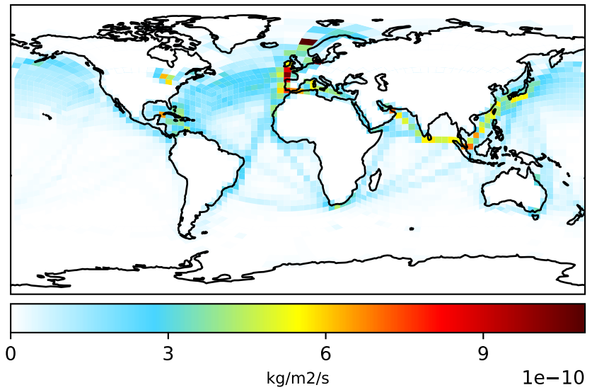
gchp_carbon-CO2 (Dev) c24
