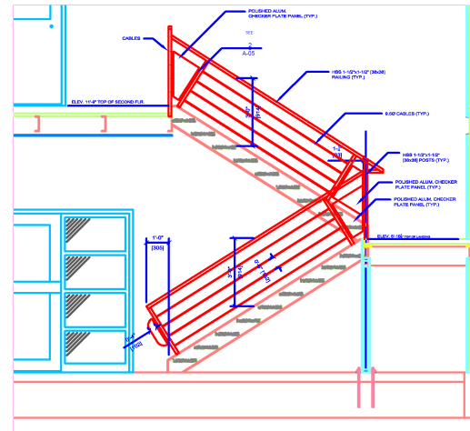
1 STAIR DETAIL 1 Scale: 1/2" = 1'-0"
