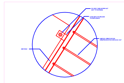
2 STAIR DETAIL 2 Scale: 3" = 1'-0"
