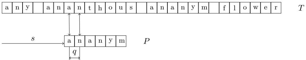
(b) 比较的起始位置移动到 s = 4 + 2 = 6 。
