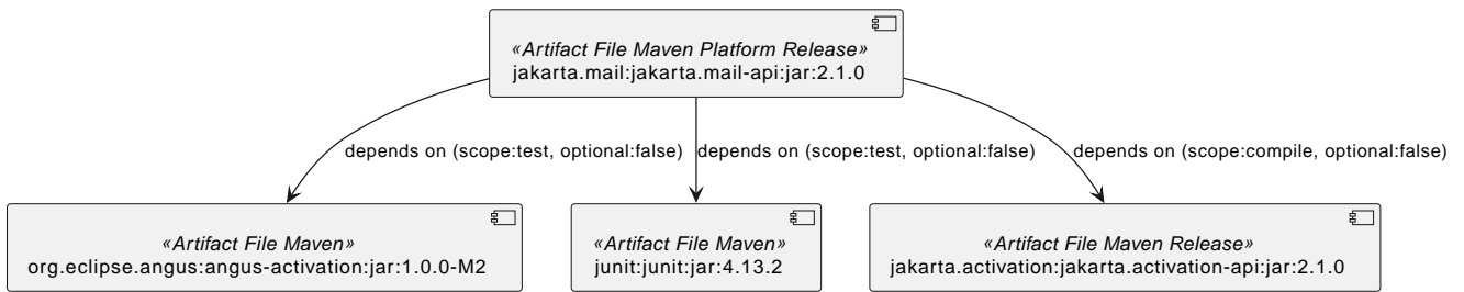
Figure 42. Jakarta Mail API 2.1.0 actual
