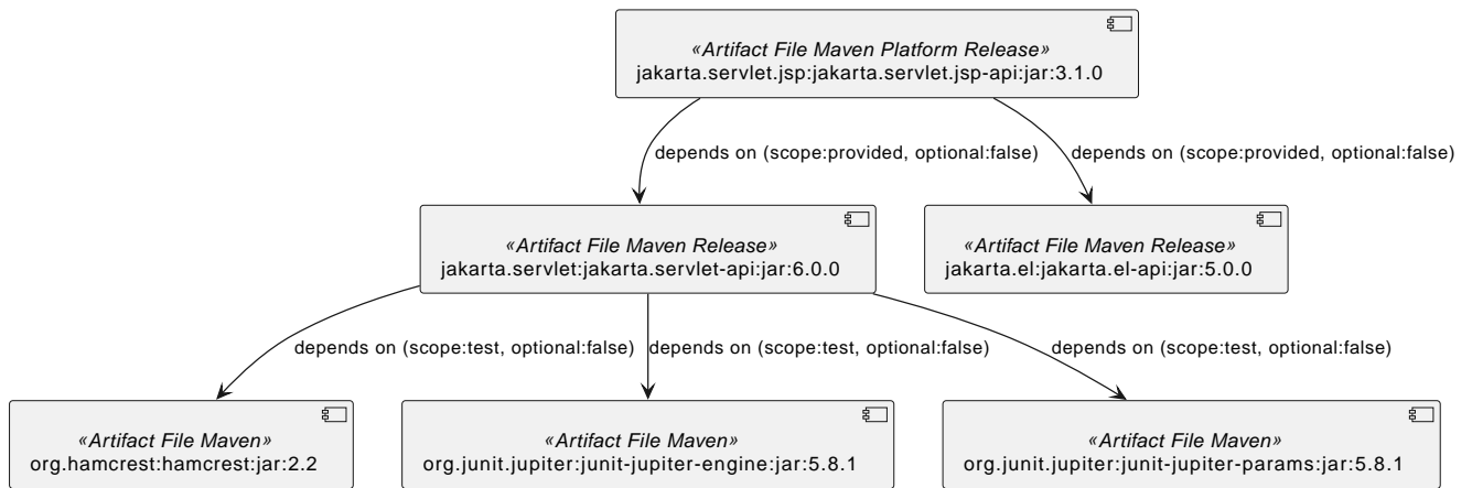
Figure 46. Jakarta Servlet JSP API 3.1.0 actual
