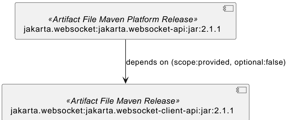
Figure 58. Jakarta Websocket (Server) API 2.1.1 actual
