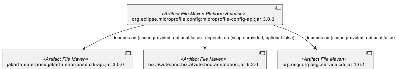
Figure 82. MicroProfile Config API 3.0.3 actual
