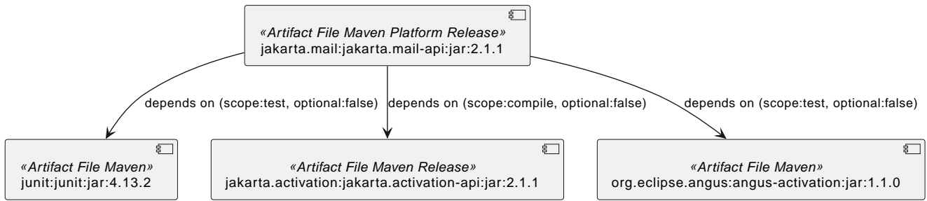
Figure 43. Jakarta Mail API 2.1.1 actual
