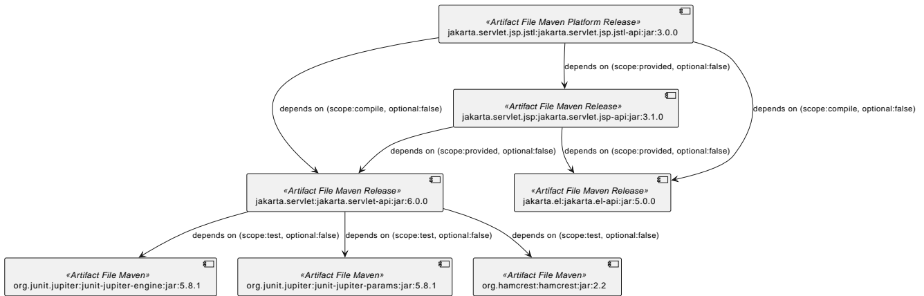
Figure 48. Jakarta Servlet JSP JSTL API 3.0.0 actual
