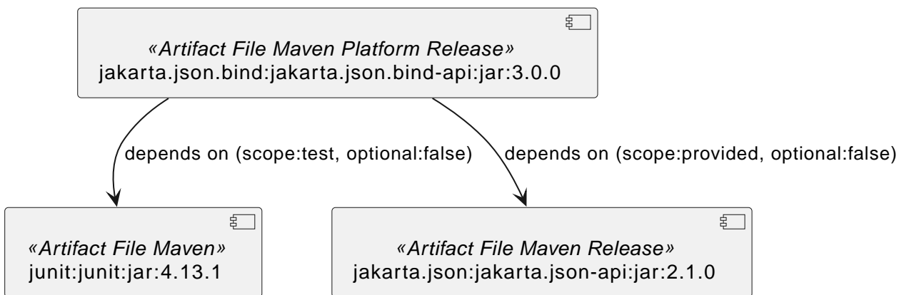
Figure 40. Jakarta JSON Bind API 3.0.0 actual
