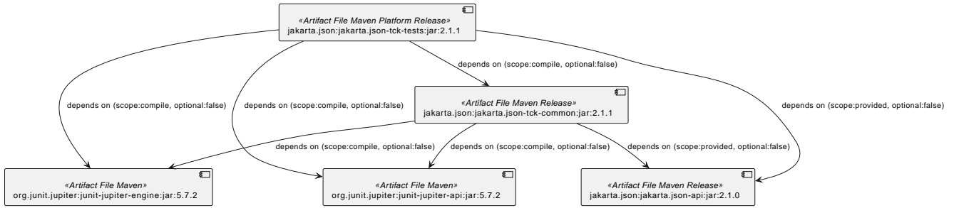
Figure 38. Jakarta JSON TCK Tests 2.1.1 actual
