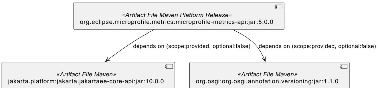
Figure 90. MicroProfile Metrics API 5.0.0 actual
