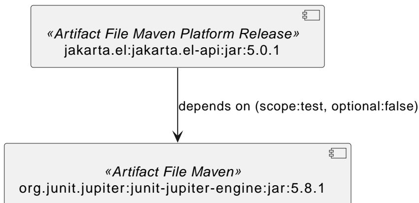
Figure 34. Jakarta EL API 5.0.1 actual
