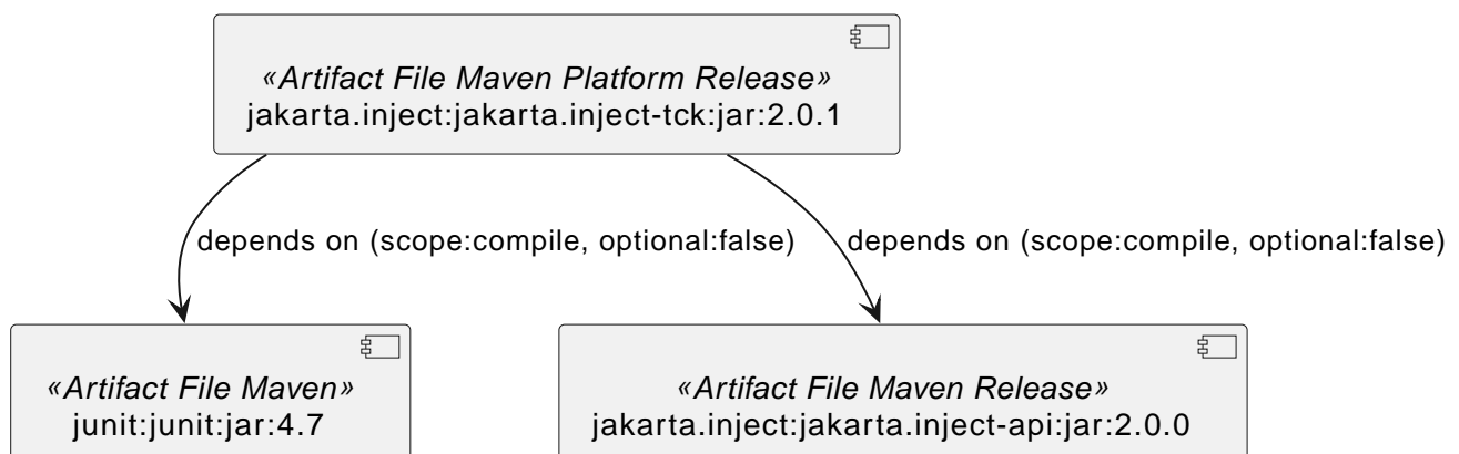
Figure 32. Jakarta Inject TCK 2.0.1 actual
