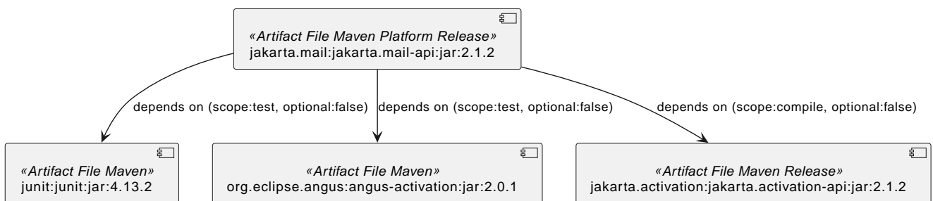
Figure 44. Jakarta Mail API 2.1.2 actual
