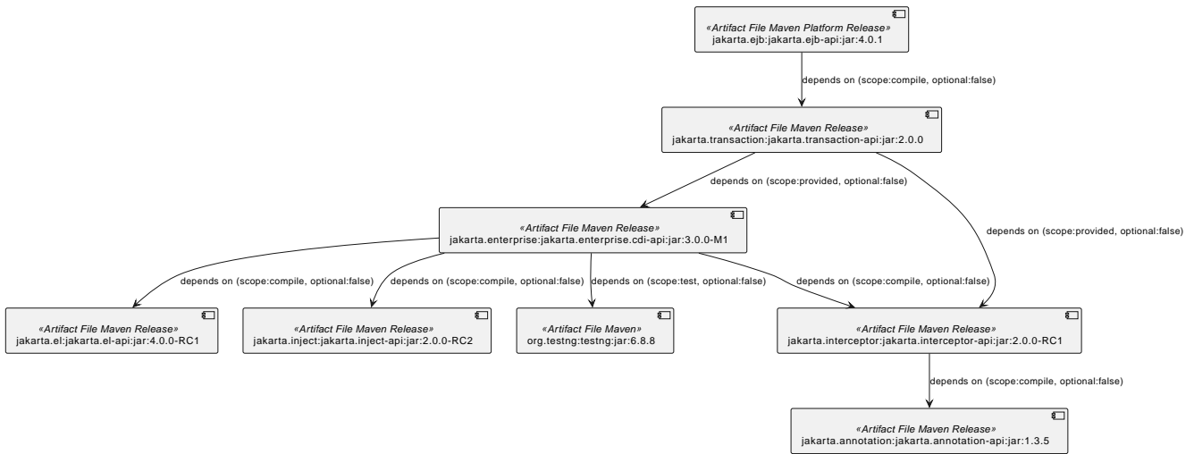
Figure 33. Jakarta EJB API 4.0.1 actual
