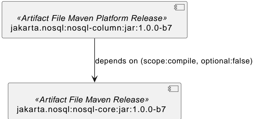
Figure 74. Jakarta NoSQL API Column 1.0.0-b7 actual
