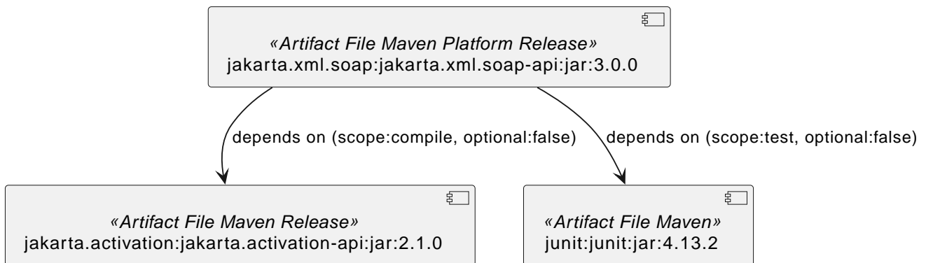
Figure 61. Jakarta XML SOAP API 3.0.0 actual
