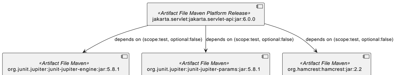
Figure 47. Jakarta Servlet API 6.0.0 actual
