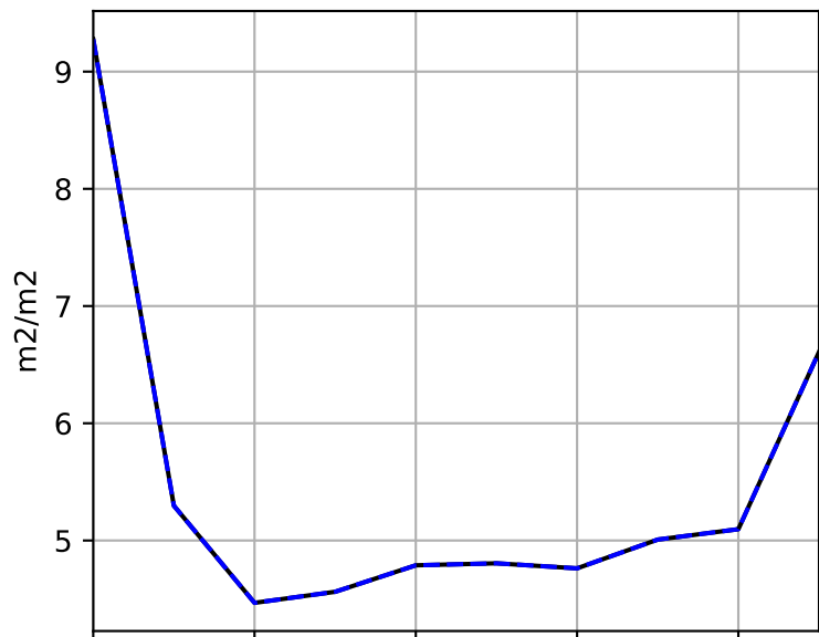
TLAI
