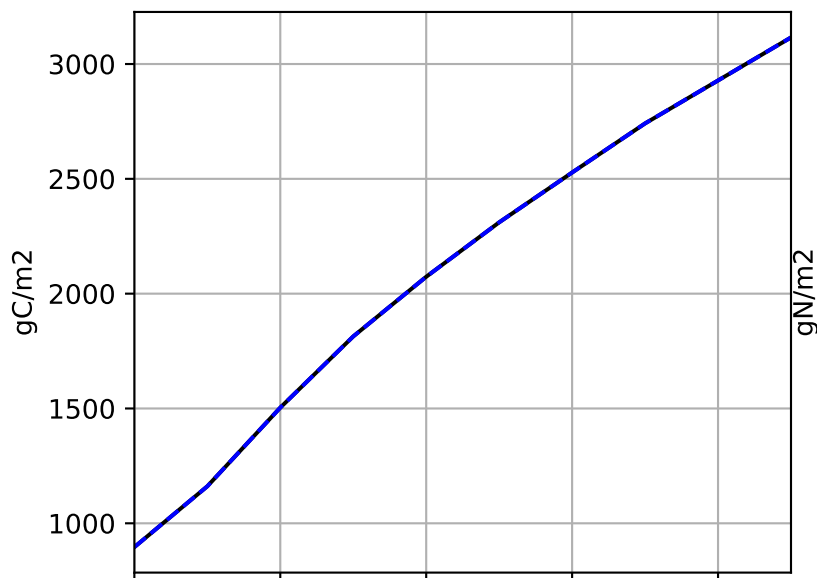
TOTSOMC
