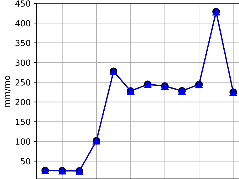
RAIN
