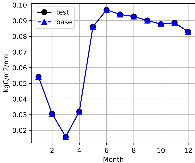
HR
