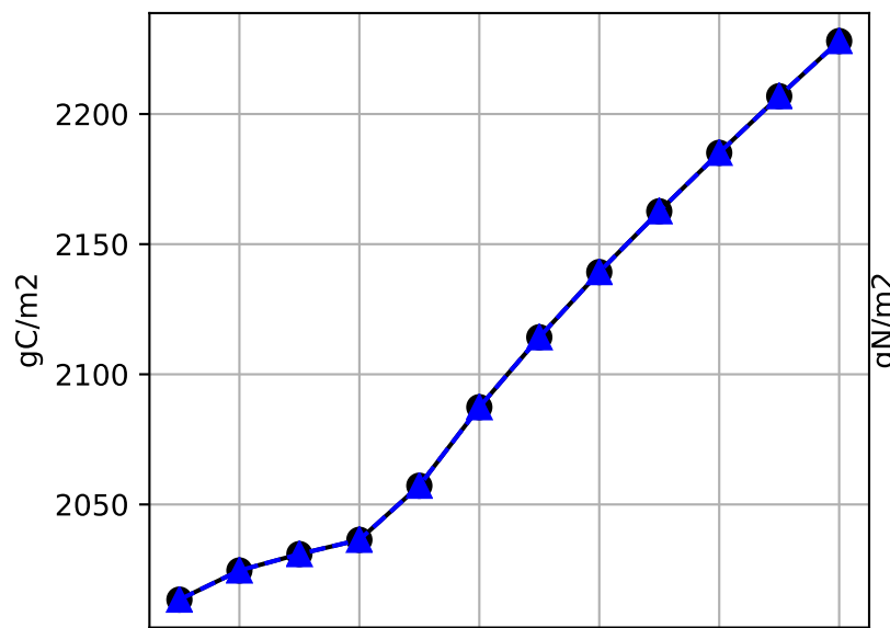
TOTSOMC
