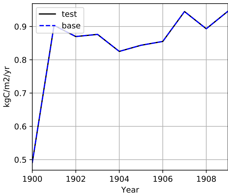
HR
