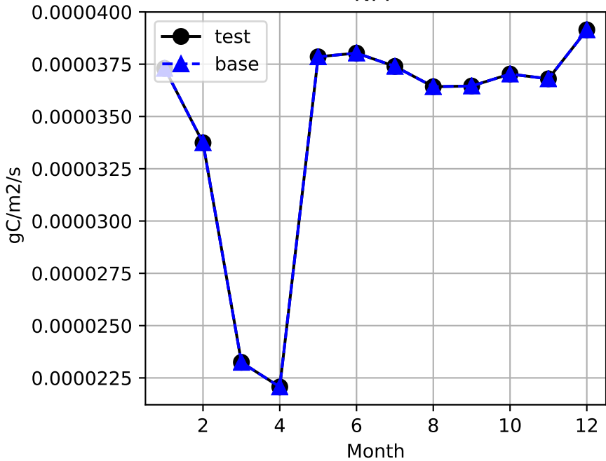
NPP
