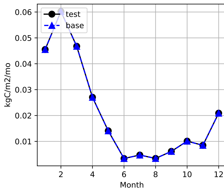
NEP
