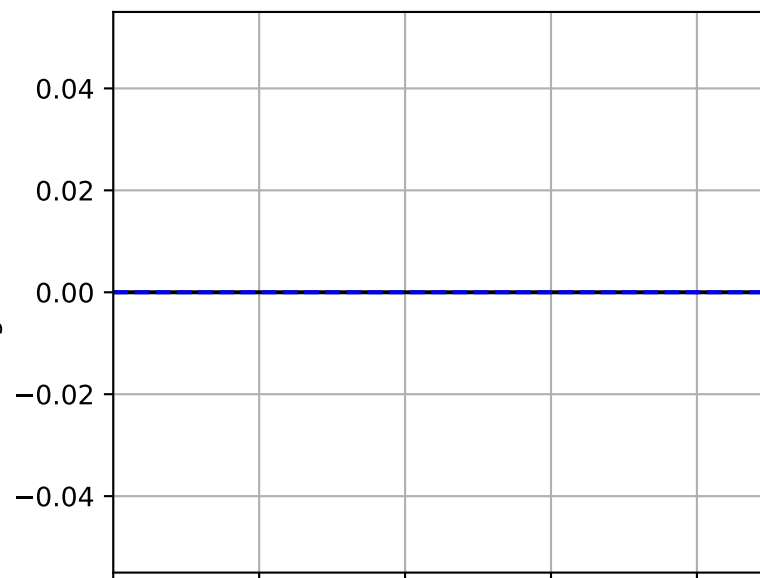
TOTSOMN
