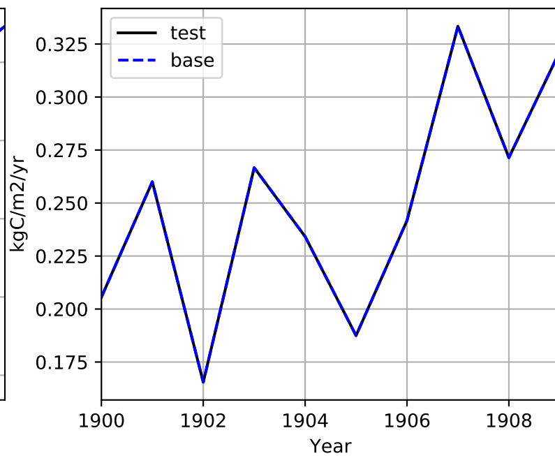
NEP
