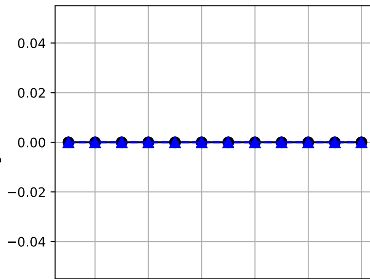
TOTSOMN
