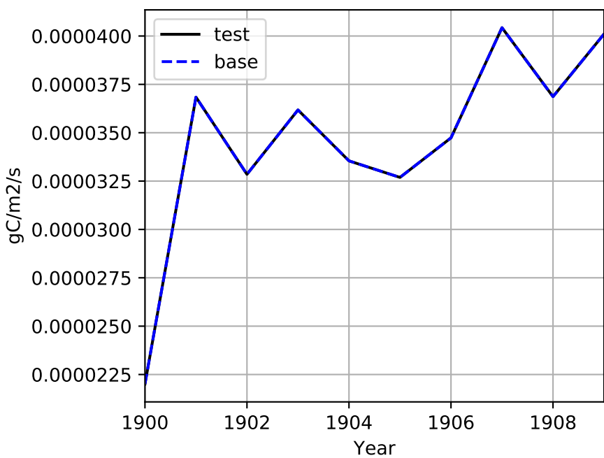
NPP
