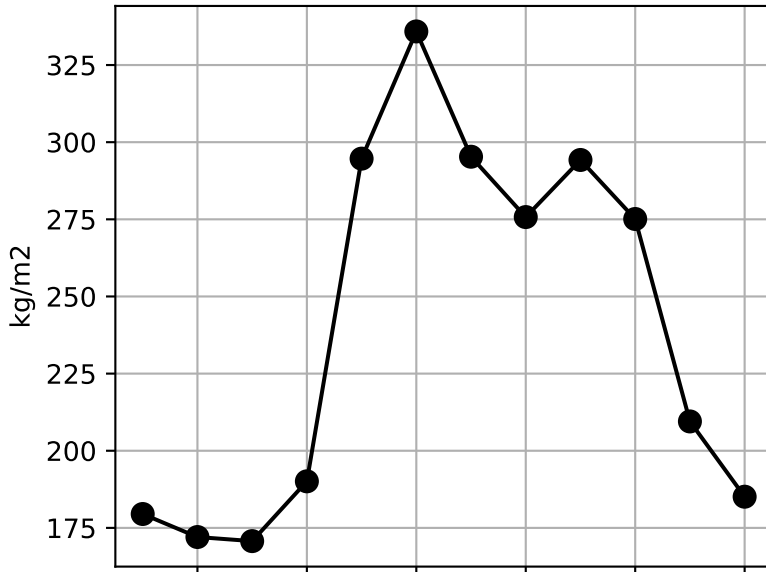
TOTSOILLIQ
