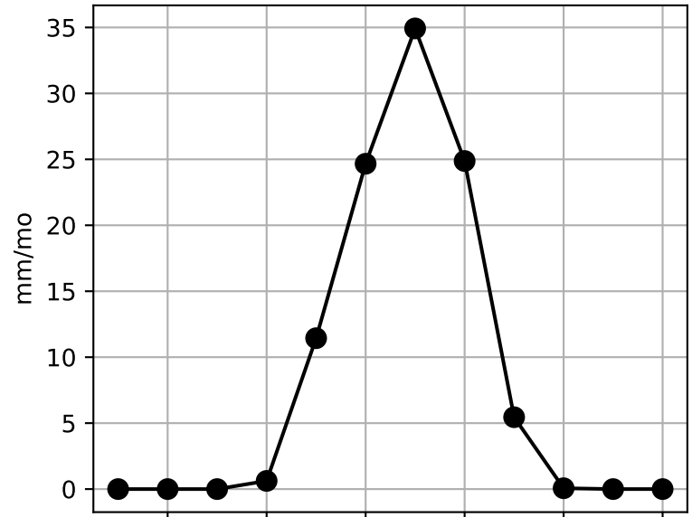
QVEGT
