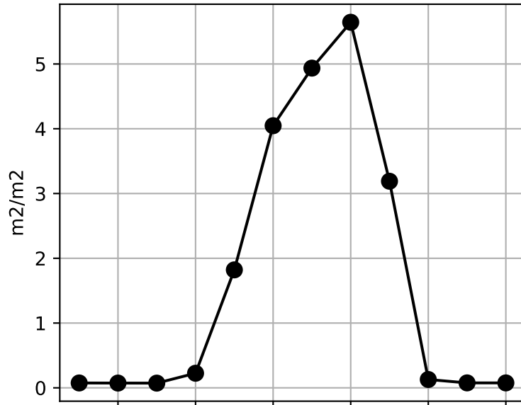
TLAI
