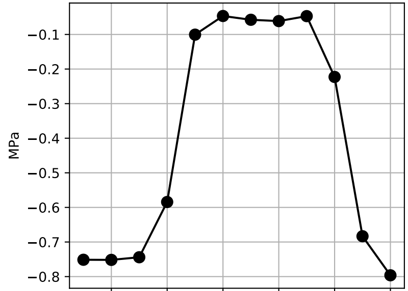
FATES_LWP_COL_SCPF
