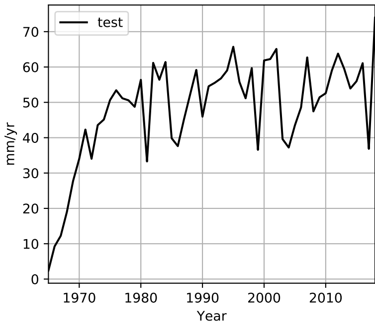
QVEGE
