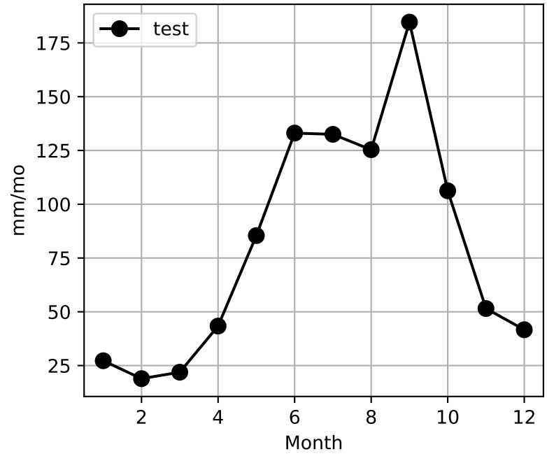
RAIN
