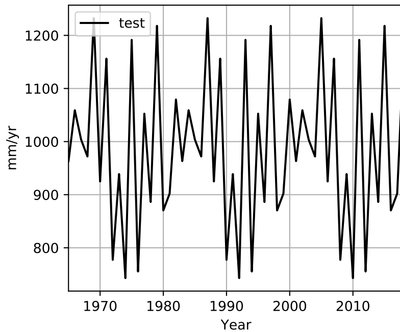
RAIN
