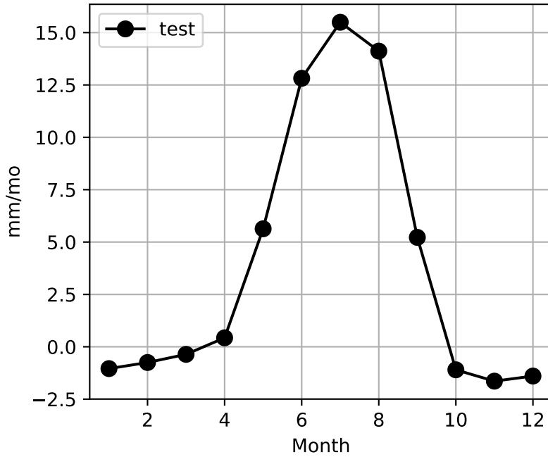
QVEGE
