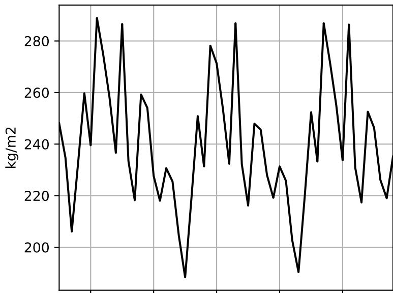
TOTSOILLIQ
