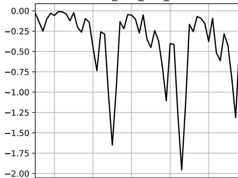
FATES_LWP_COL_SCPF
