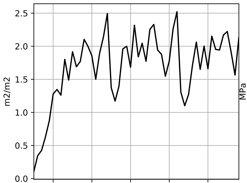
TLAI
