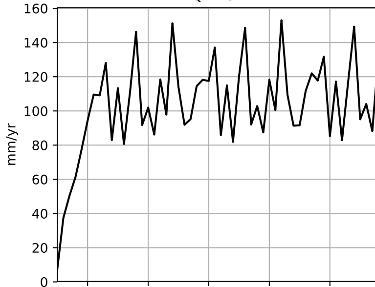
QVEGT
