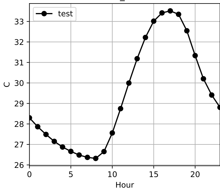
TSOI_10CM
