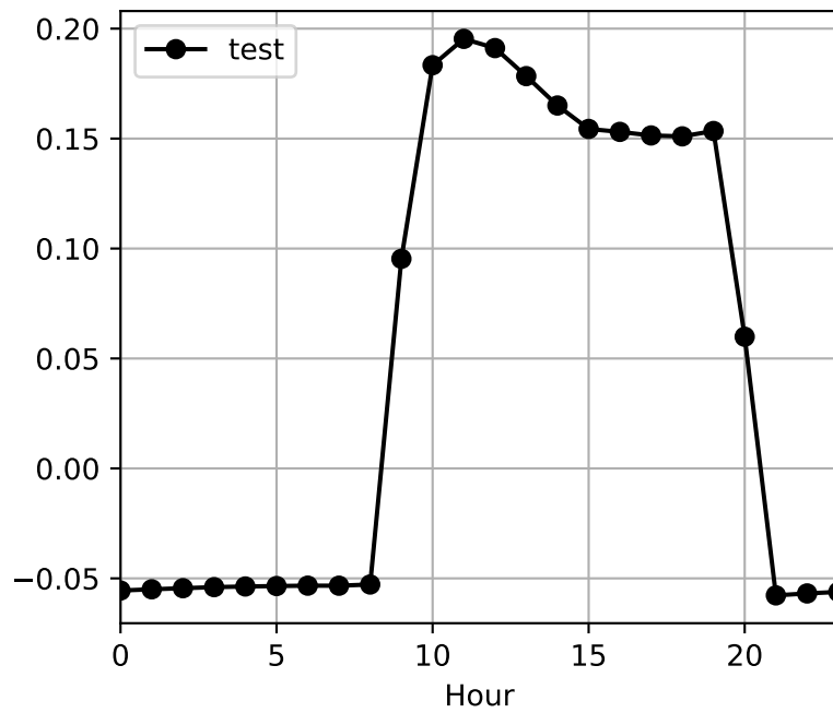
NPP
