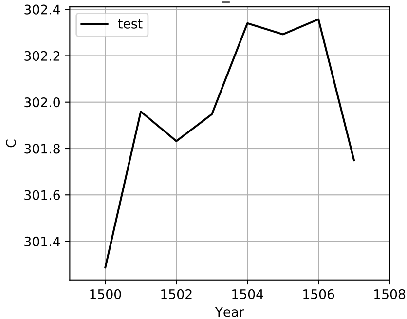
TSOI_10CM
