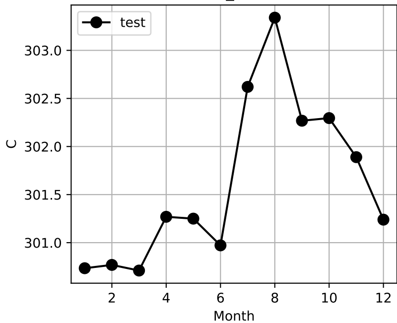
TSOI_10CM
