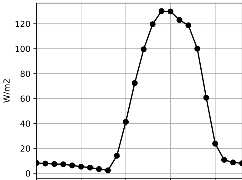
FSH
