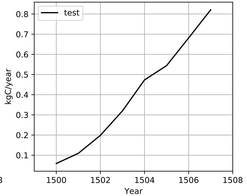
NPP
