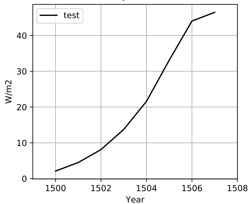
QVEGT
