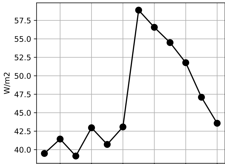
FSH
