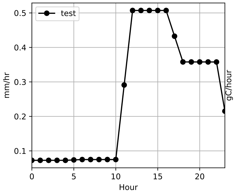
RAIN
