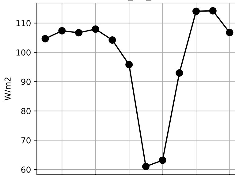
EFLX_LH_TOT
