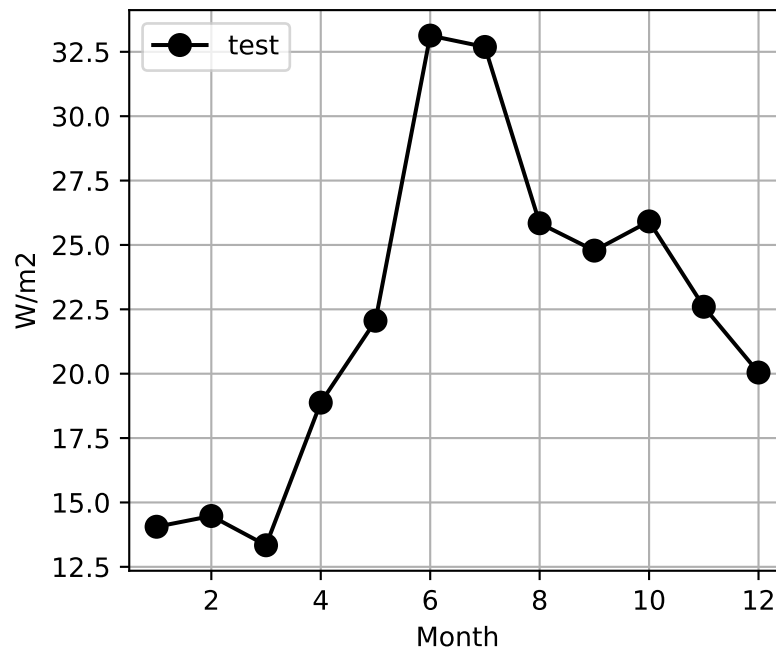
QVEGT
